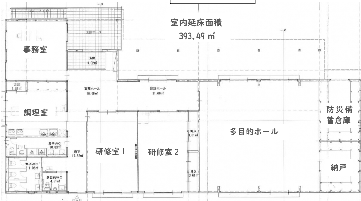
要望調整平面図
