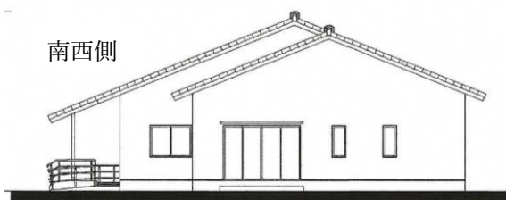
新交流センター立面図
