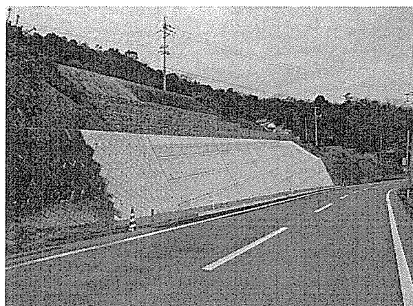
平成25年災 那賀東部広域農道災害復旧工事(その1)
