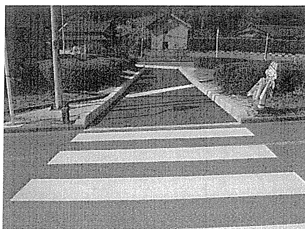
平成25年度市道小田1号線歩道設置工事
