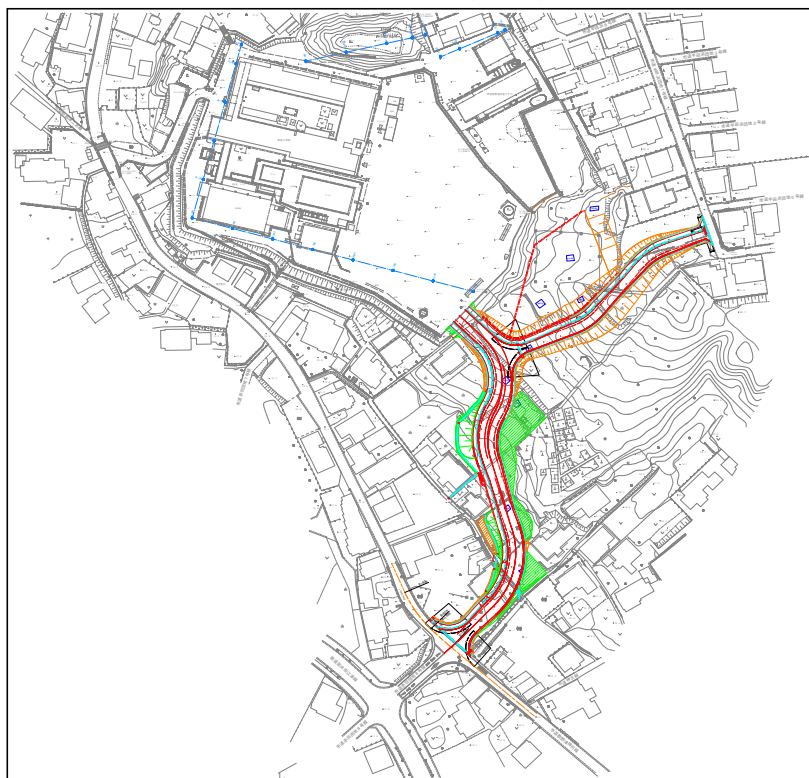
市道赤羽根団地8号線測量設計業務（計画平面図）
