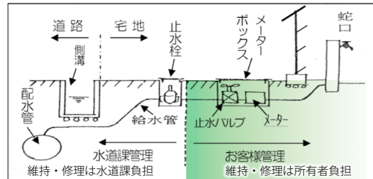
水道管の管理区分図
