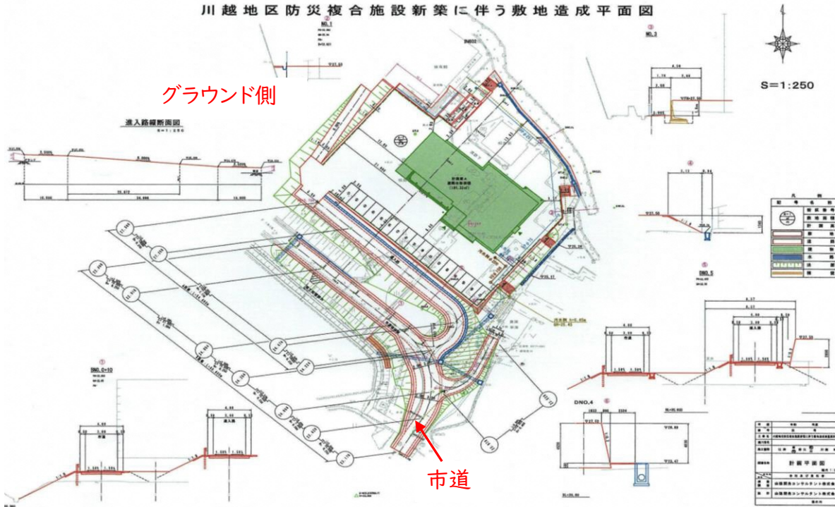
川越地区防災複合施設新築に伴う敷地造成平面図
